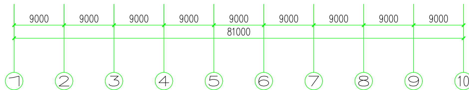
±0.00平面布置图 1:500
